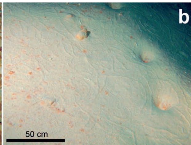
Figure 42: a) Vermiculacions made up of reddish siliceous silty sediments. b) Vermiculacions of carbonate sediments. Endavant les Atxes gallery. (Photo F. Gràcia).
