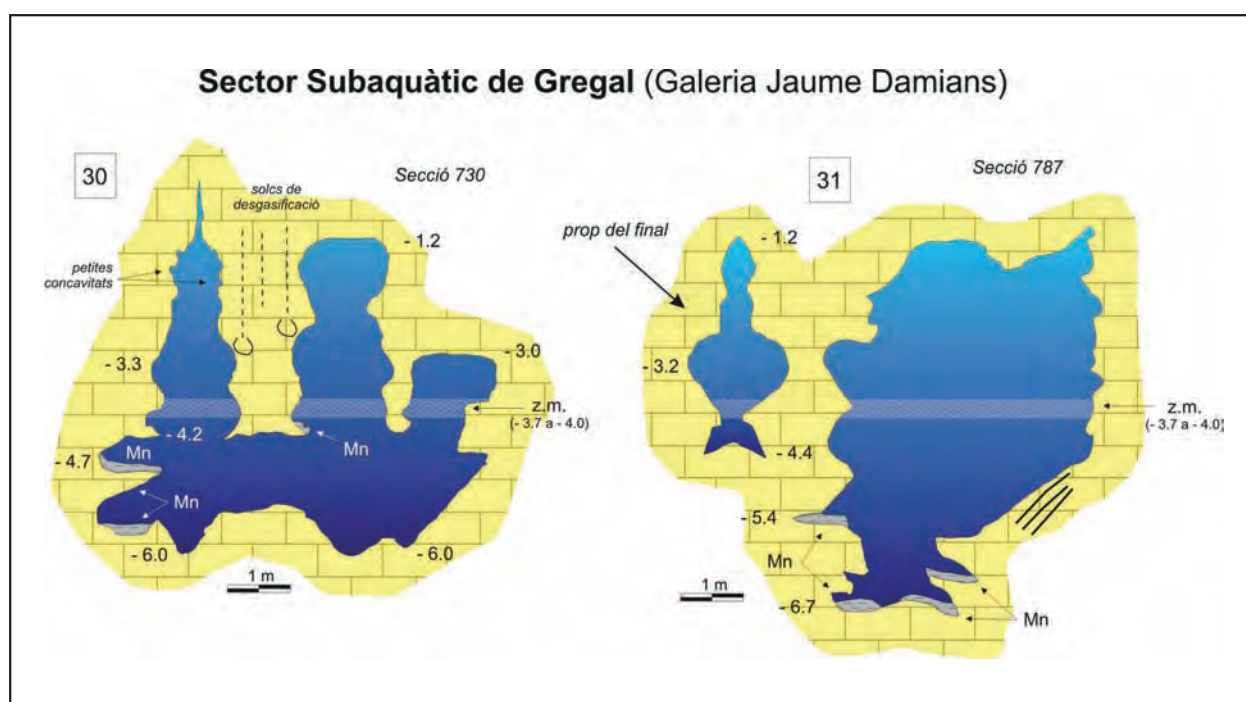
Figura 23: Seccions de la galeria Jaume Damians.
