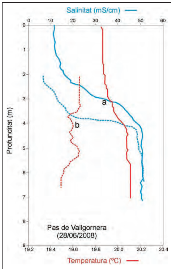
Figura 27: Perfil hídric de dues localitzacions de la cavitat. a) Branca Oriental del sector Antic, entre 0 i -7 m; b) Galeria Collonuda Nord (sector Subaquàtic de Gregal), entre -2,5 i -7 m.
